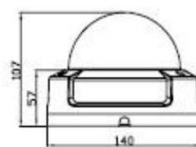
防爆半球外形尺寸
