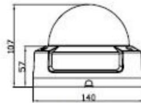
防爆半球外形尺寸
